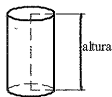
Cilindro recto
