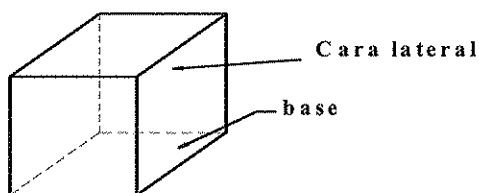
Poliedro convexo
