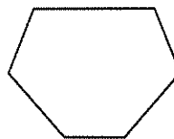
polígono convexo no regular
