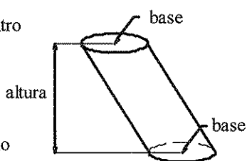
Cilindro oblicuo
