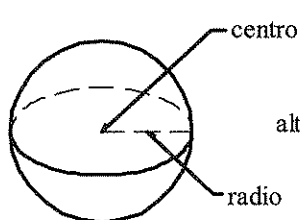
Esfera
