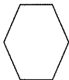
polígono convexo regular
