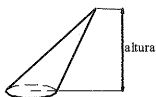
Cono oblicuo
