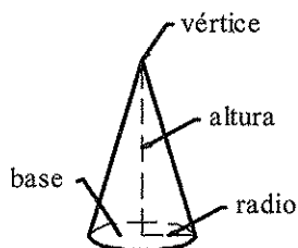
Cono
